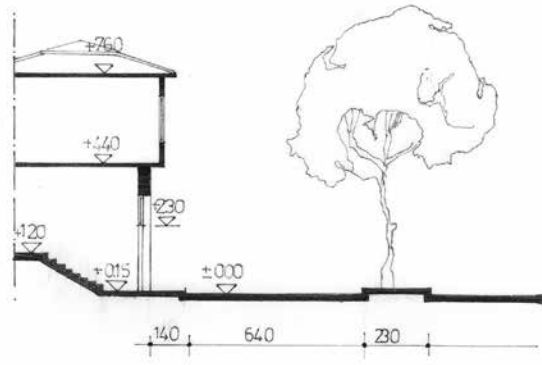
A-A KESİTİ
