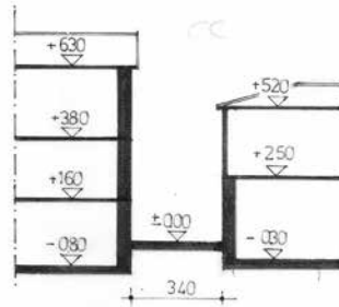
C-C KESİTİ
