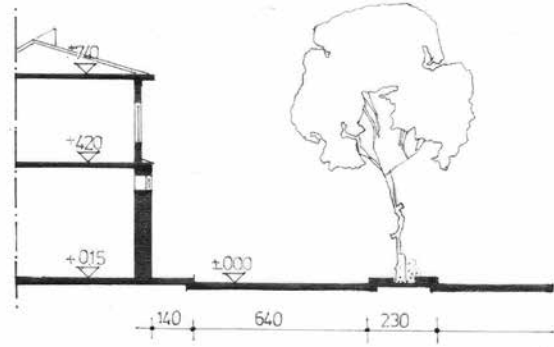
C-C KESİTİ
