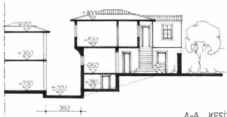
A-A KESİTİ
