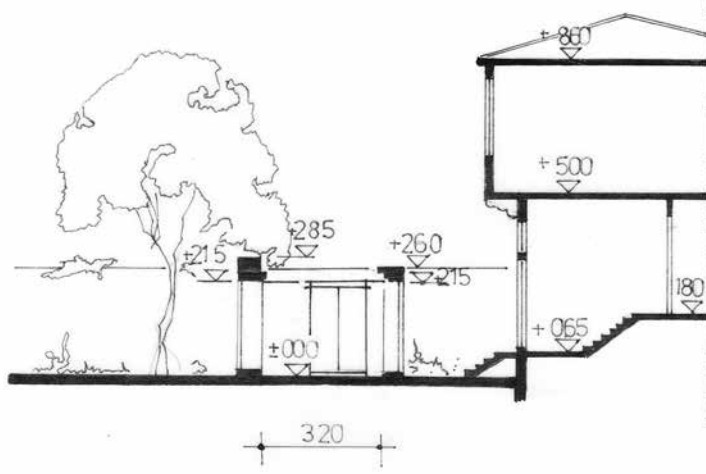
A-A KESİTİ
