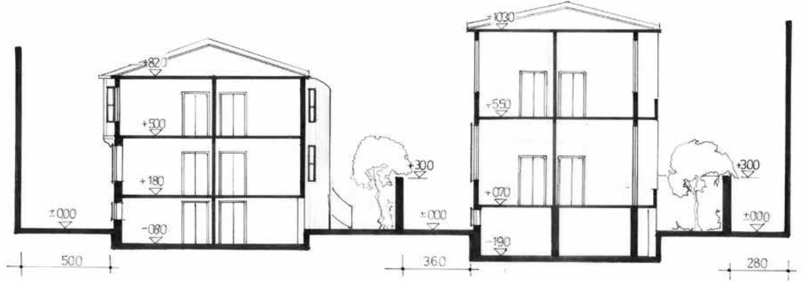
A-A KESİTİ
