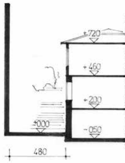
A-A KESİTİ
