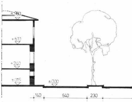
B-B KESİTİ
