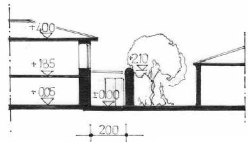
G-C KESİTİ
