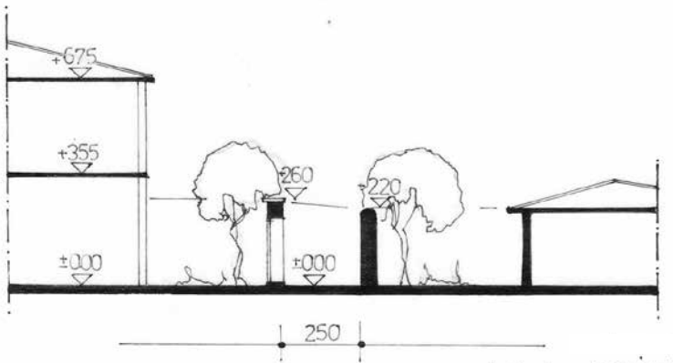
A-A KESİTİ
