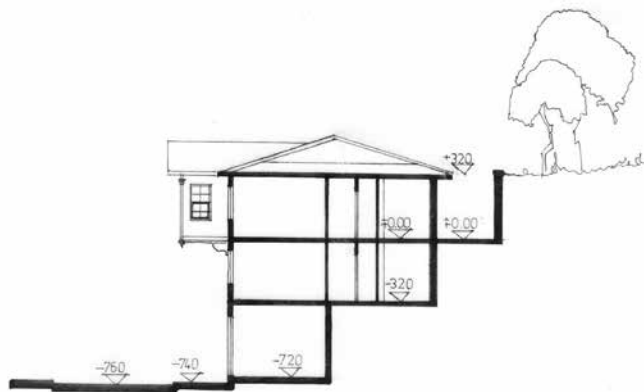
A-A KESİTİ
