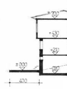
D D KESİTİ
